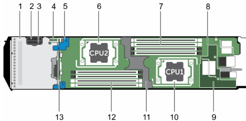
Abbildung 9. Das Innere des Schlittens
