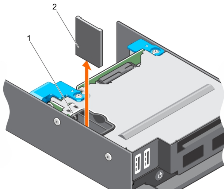
Abbildung 22. Austauschen der vFlash SD-Karte
