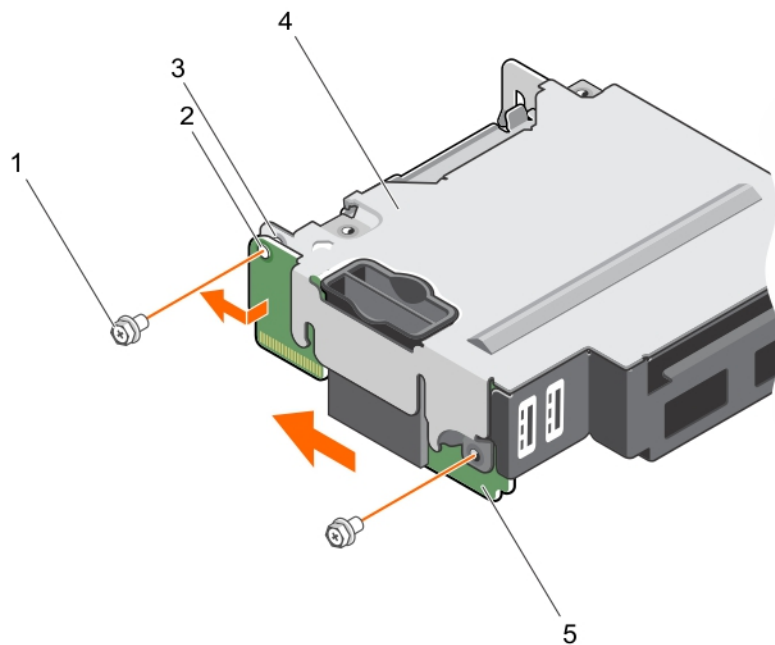
Abbildung 20. Entfernen der IDSDM-Karte
