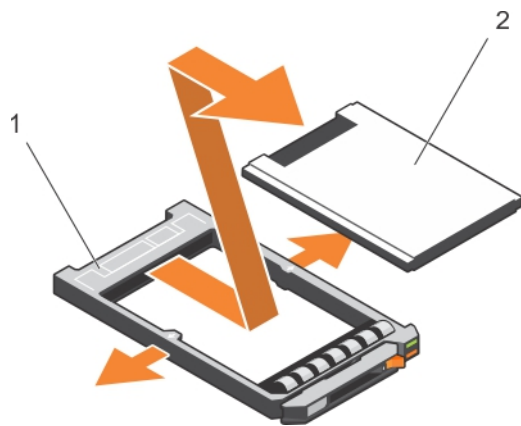
Abbildung 32. Entfernen eines SSD-Laufwerks aus einem SSD-Träger
