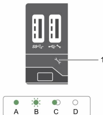
Abbildung 5. iDRAC Direct-LED-Anzeige
