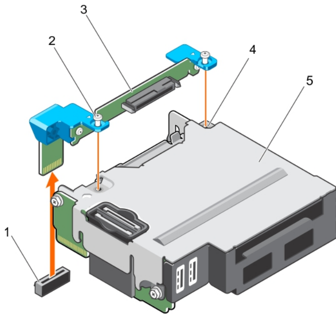
Abbildung 40. Entfernen der SSD-Rückwandplatine
