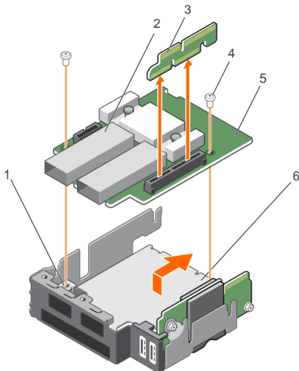
Abbildung 16. Entfernen einer PCIe-Zusatzkarte
