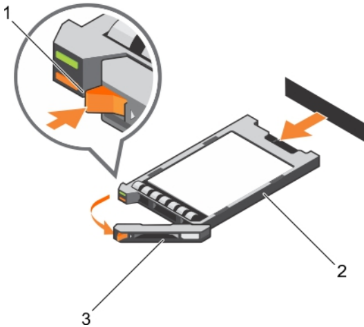
Abbildung 34. Entfernen eines SSD-Trägers
