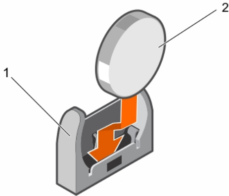
Abbildung 43. Installieren der NVRAM-Stützbatterie
