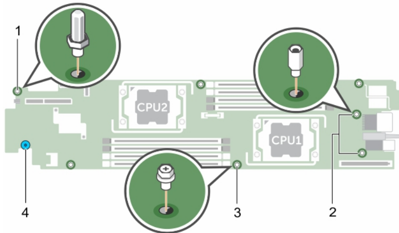
Abbildung 44. Position der Schraube auf der Systemplatine
