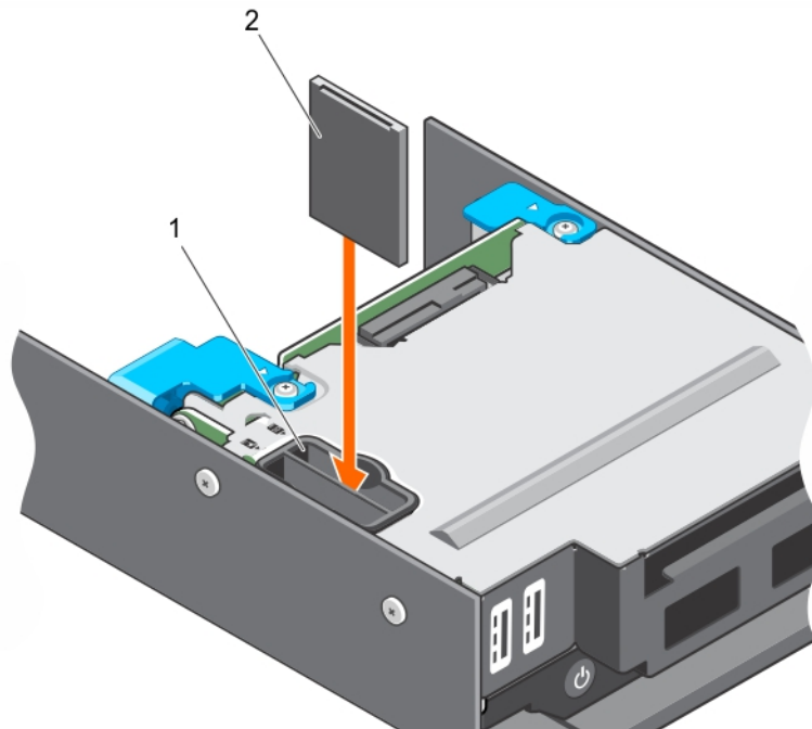
Abbildung 19. Einsetzen einer internen SD-Karte
