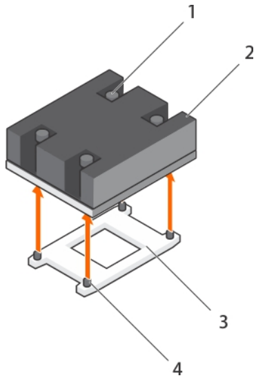
Abbildung 26. Entfernen des 120-W-Kühlkörpers
