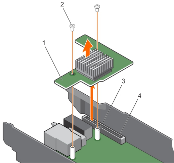
Abbildung 24. Entfernen der LOM-Riser-Karte
