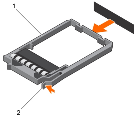
Abbildung 36. Entfernen eines Laufwerkplatzhalters
