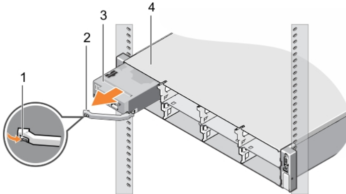
Abbildung 7. Entfernen eines Schlittens
