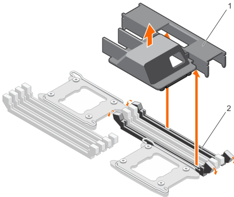
Abbildung 31. Entfernen eines Prozessor- und DIMM-Platzhalters
