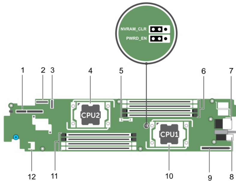
Abbildung 48. Systemplatinenanschlüsse
