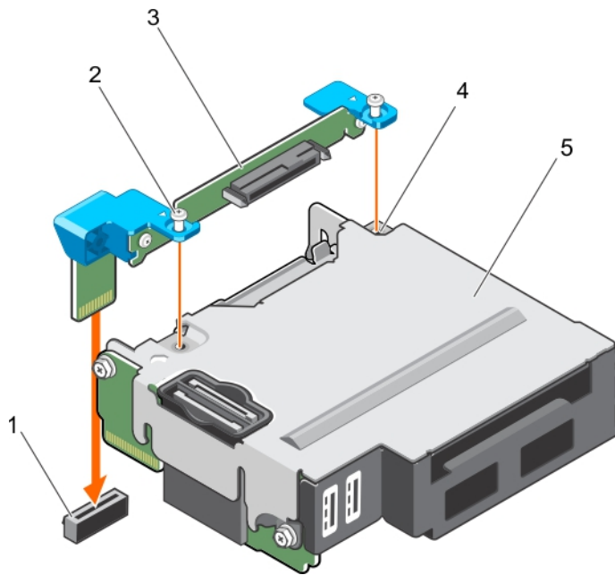
Abbildung 41. Einsetzen der SSD-Rückwandplatine
