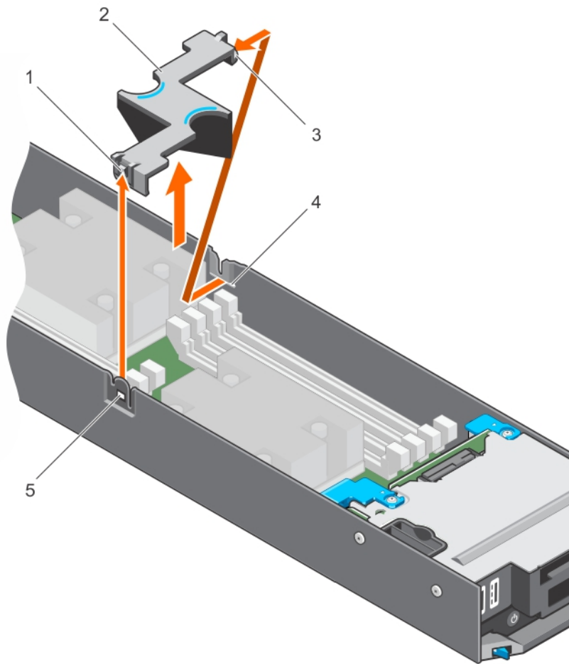
Abbildung 10. Entfernen des Kühlgehäuses
