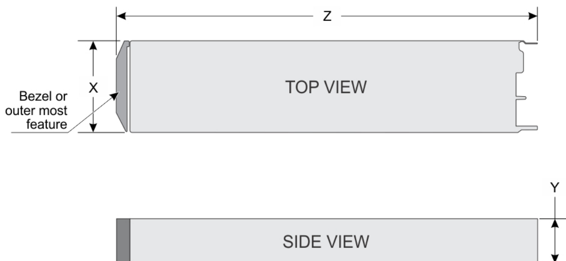
Abbildung 6. Gehäuseabmessungen des PowerEdge FC430-Systems
