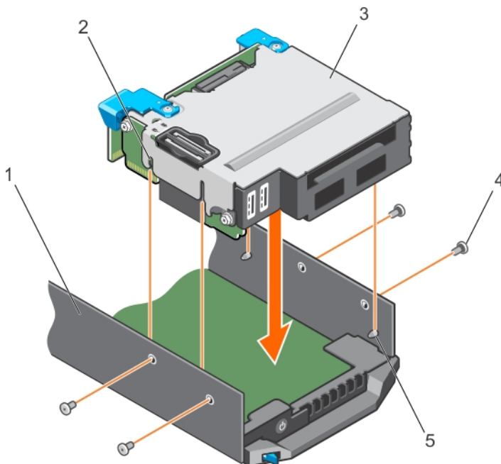
Abbildung 39. Einsetzen der SSD-Laufwerkabschirmung
