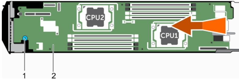
Abbildung 46. Einsetzen der Systemplatine
