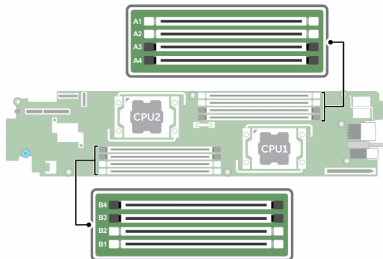
Abbildung 12. Positionen der Speichersockel
