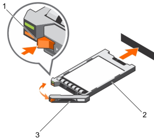
Abbildung 35. Einsetzen eines SSD-Trägers
