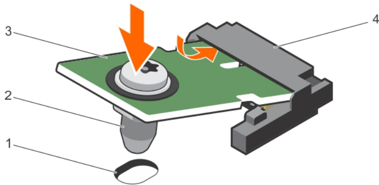
Abbildung 47. Einsetzen des TPM
