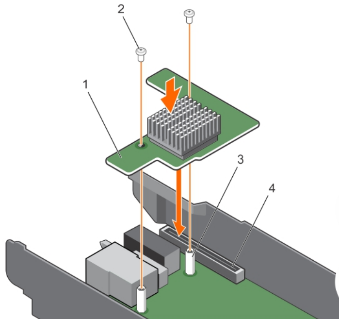
Abbildung 25. Einsetzen der LOM-Riser-Karte
