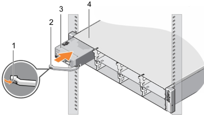
Abbildung 8. Einbauen eines Schlittens
