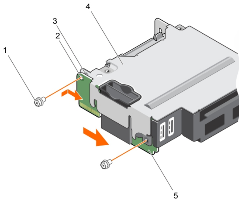
Abbildung 21. Installieren der IDSDM-Karte
