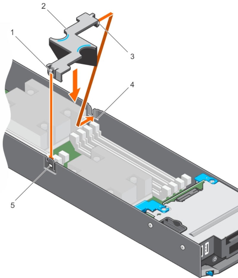
Abbildung 11. Einsetzen des Kühlgehäuses
