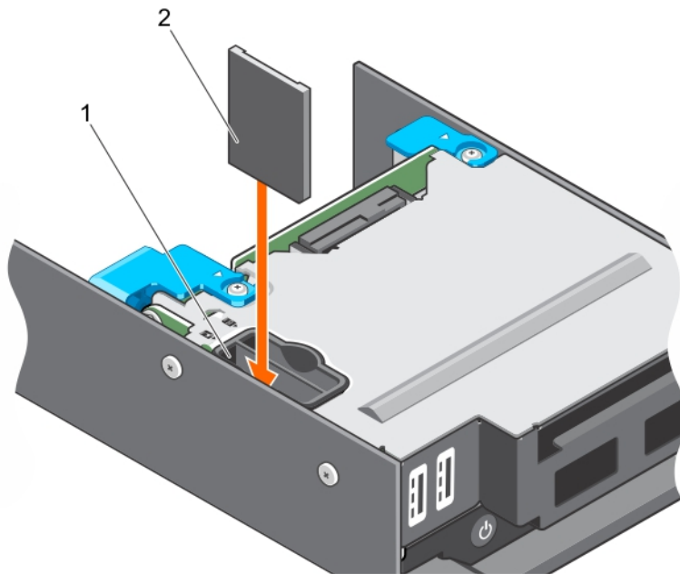
Abbildung 23. Installieren der vFlash SD-Karte
