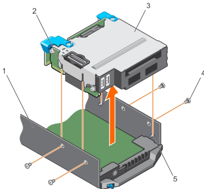
Abbildung 38. Entfernen einer SSD-Laufwerkabschirmung
