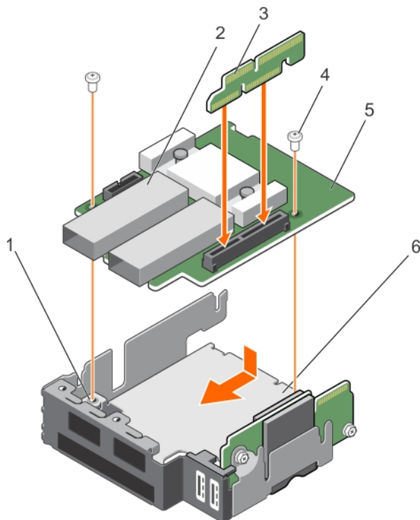
Abbildung 17. Installieren der PCIe-Zusatzkarte
