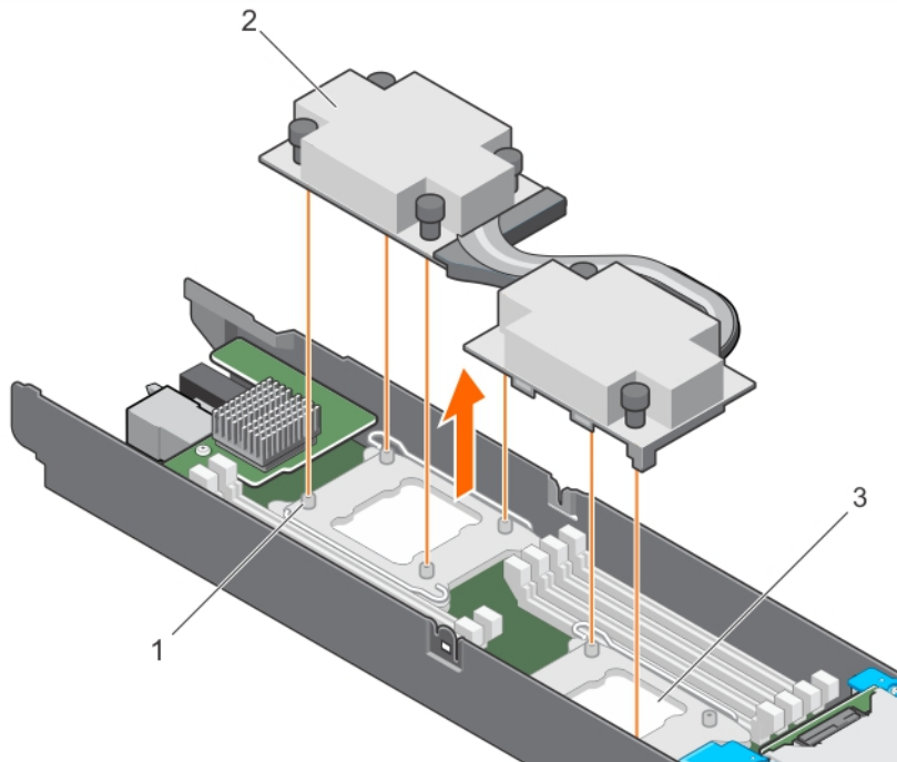
Abbildung 27. Entfernen des 140-W-Kühlkörpers
